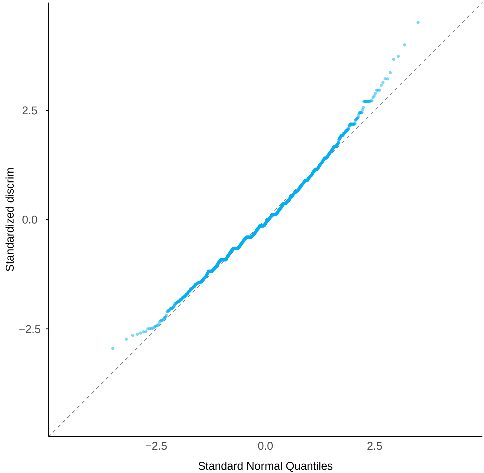
Normal Q-Q: discrim
